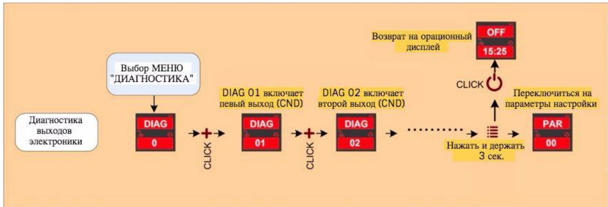
рис. 13: описание меню
