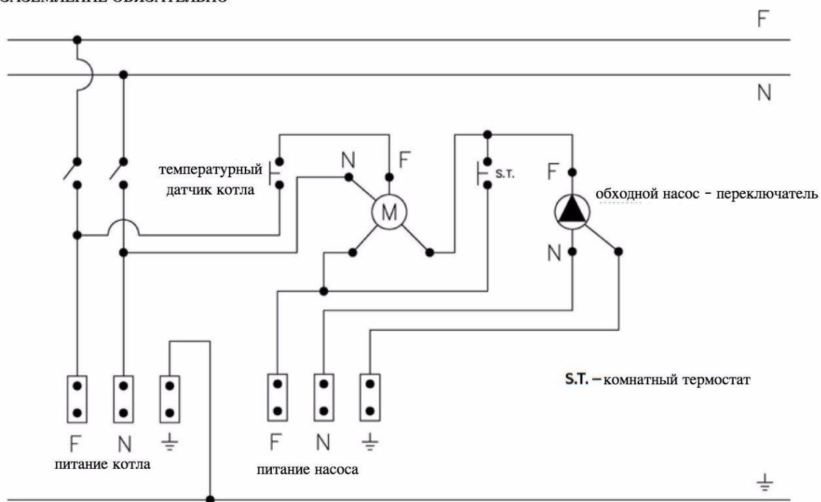
Электрическая схема 2
