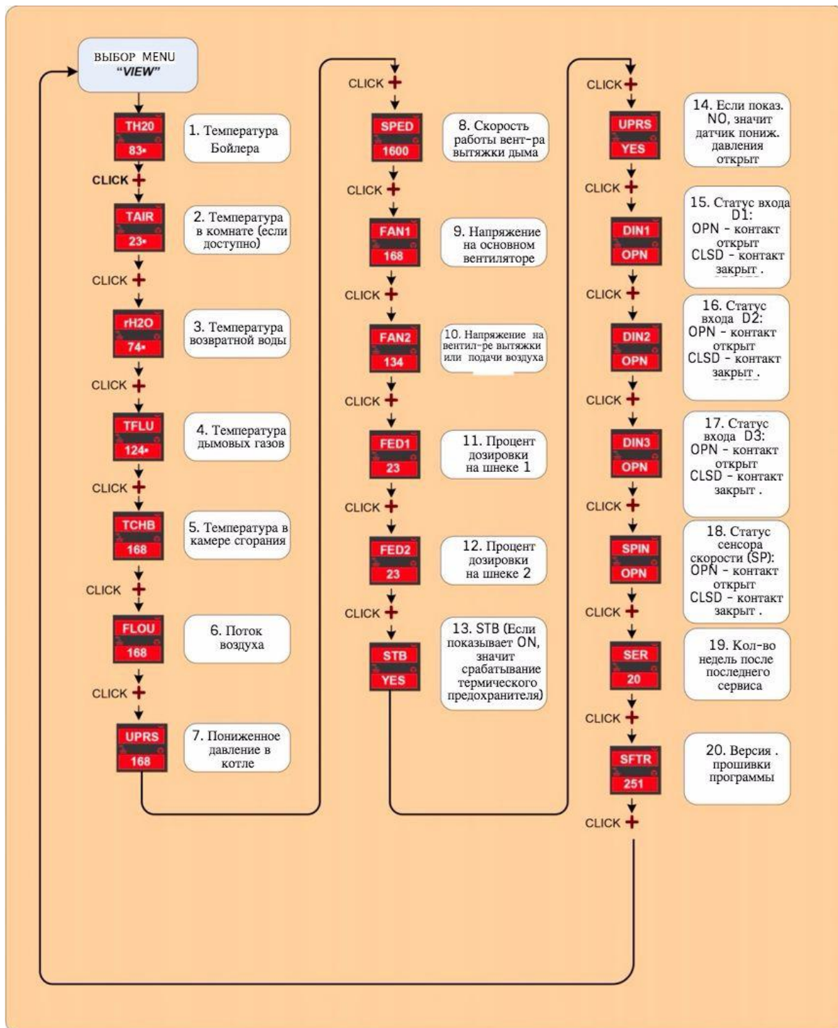
рис. 13: описание меню
